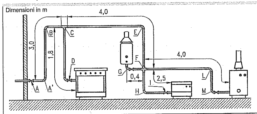
Schema di impianto interno - Determinazione dei diametri
