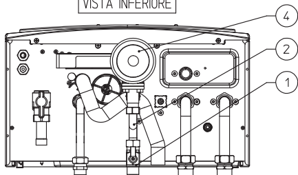
VISTA INFERIORE
