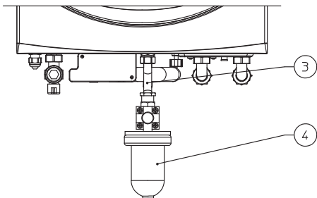
VISTA FRONTALE
