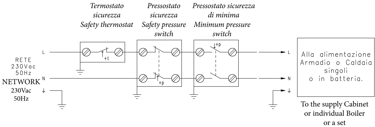
Schema elettrico per collegamento kit pressostato di minima a caldaia singola o in batteria Wiring diagram for the minimum pressure switch kit connection to a single boiler or a set
