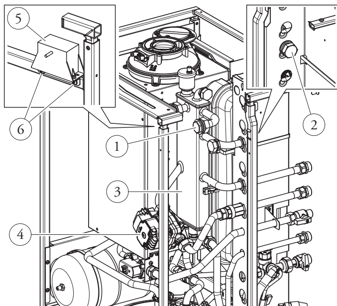
CALDAIA STANDARD
