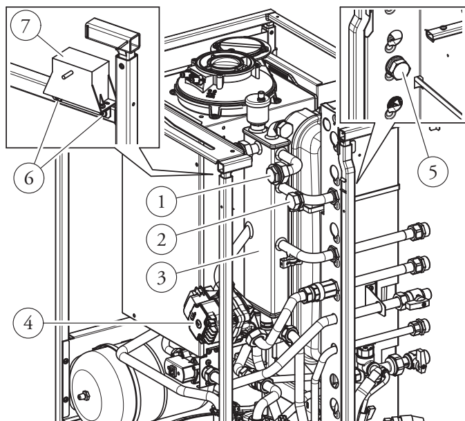
CALDAIA STANDARD
