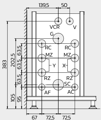
ALLACCIAMENTO LATERALE DESTRO
