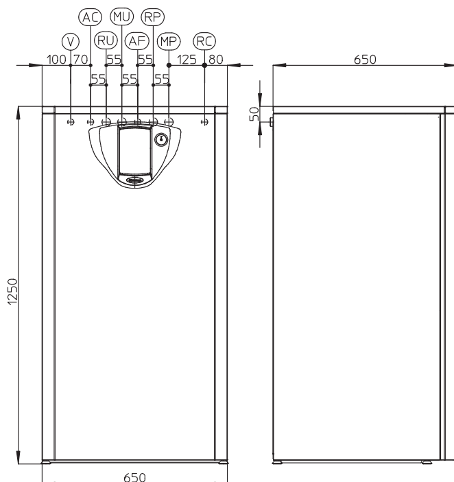
Unità bollitore Inox 200 Litri
