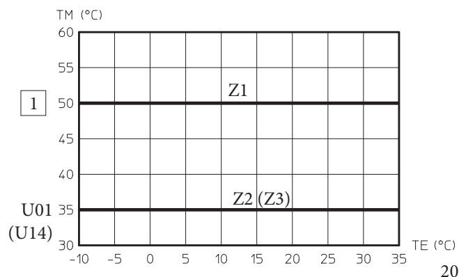
Temperatura di mandata in fase riscaldamento senza sonda esterna
