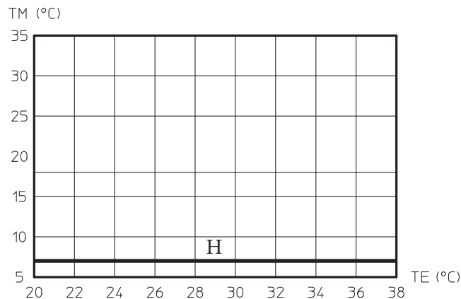
Temperatura di mandata di zona in fase raffrescamento e modulazione sonda esterna assente
