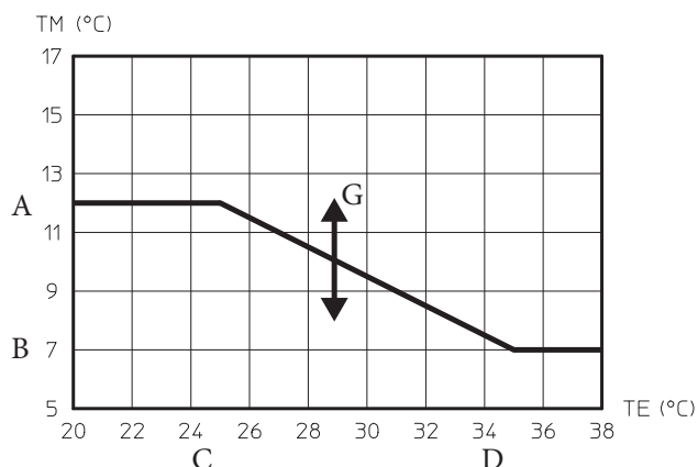
Temperatura di mandata di zona in fase raffrescamento e modulazione sonda esterna abilitata
