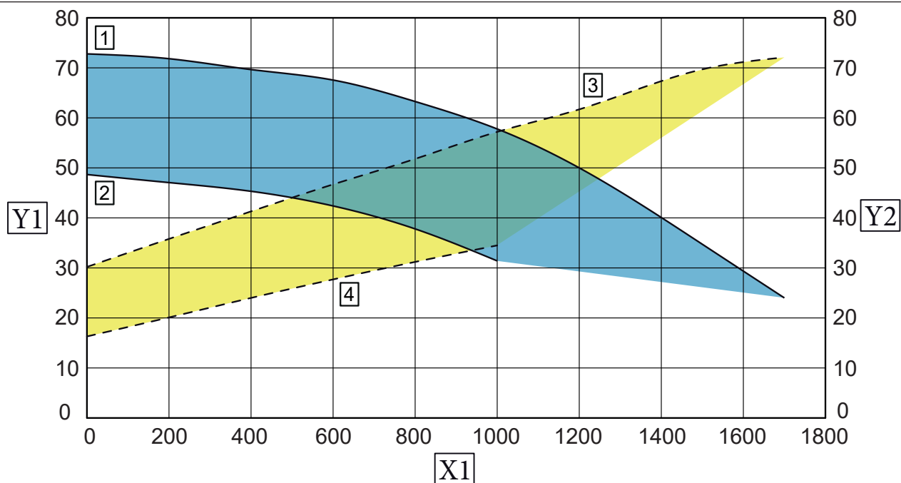
Victrix Pro 35 V2 (GRUNDFOS UPM4L)
