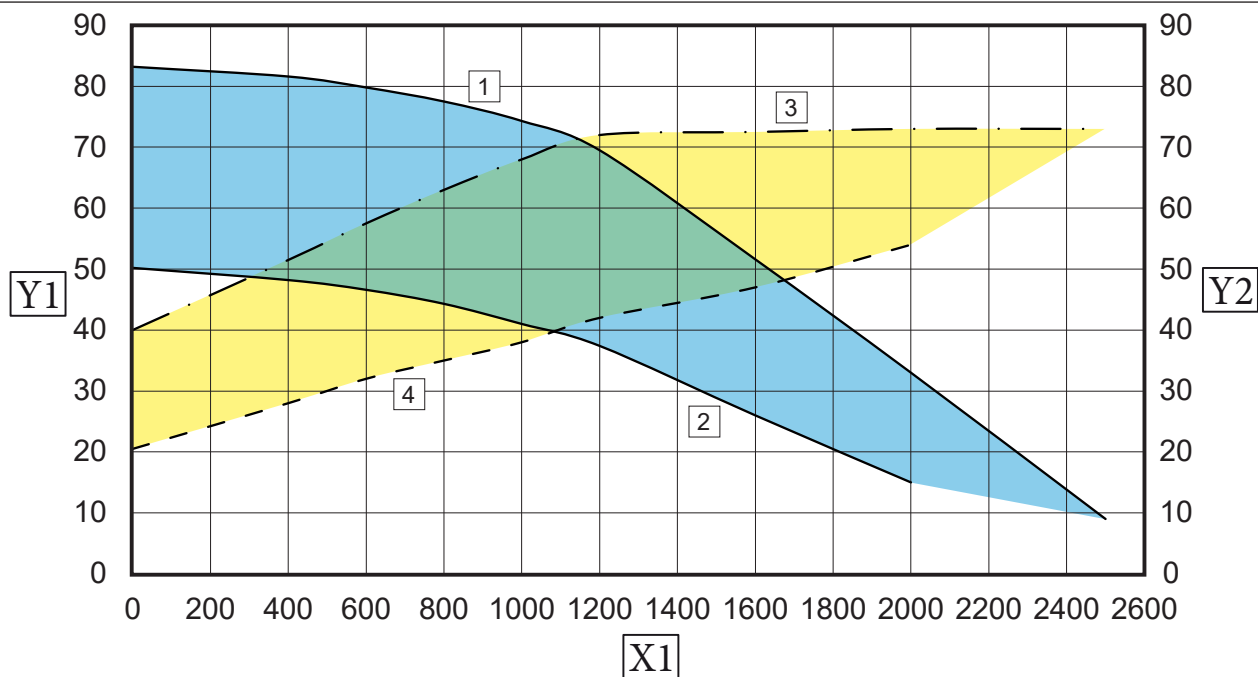
Victrix Pro 55 V2 (WILO PARA)
