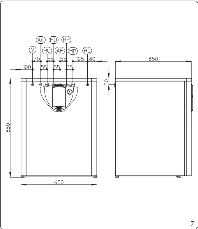
Unità bollitore Inox 120 Litri
