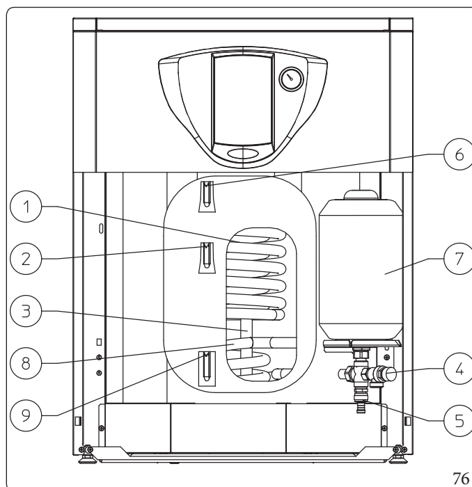
Unità bollitore Inox 120 Litri
