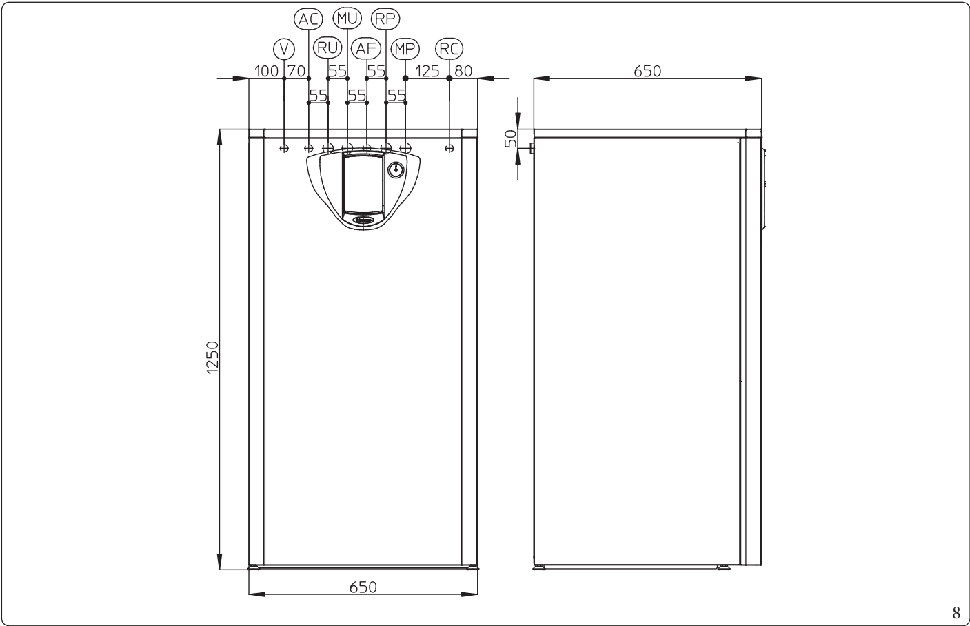
Unità bollitore Inox 200 Litri
