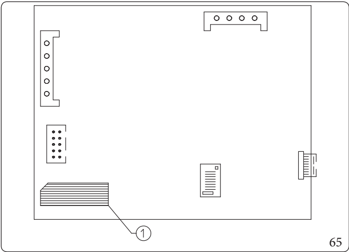
Legenda (Fig. 65): 1 - Memoria estraibile di colore nero (A19)
