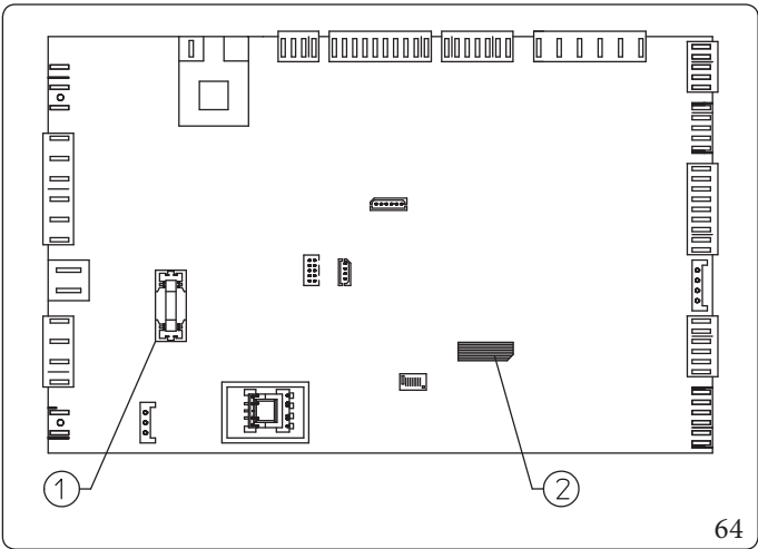
Legenda (Fig. 64): 1 - Fusibile 3,15 A rapido 250 V Tipo F 2 - Memoria estraibile di colore grigio (A19)
