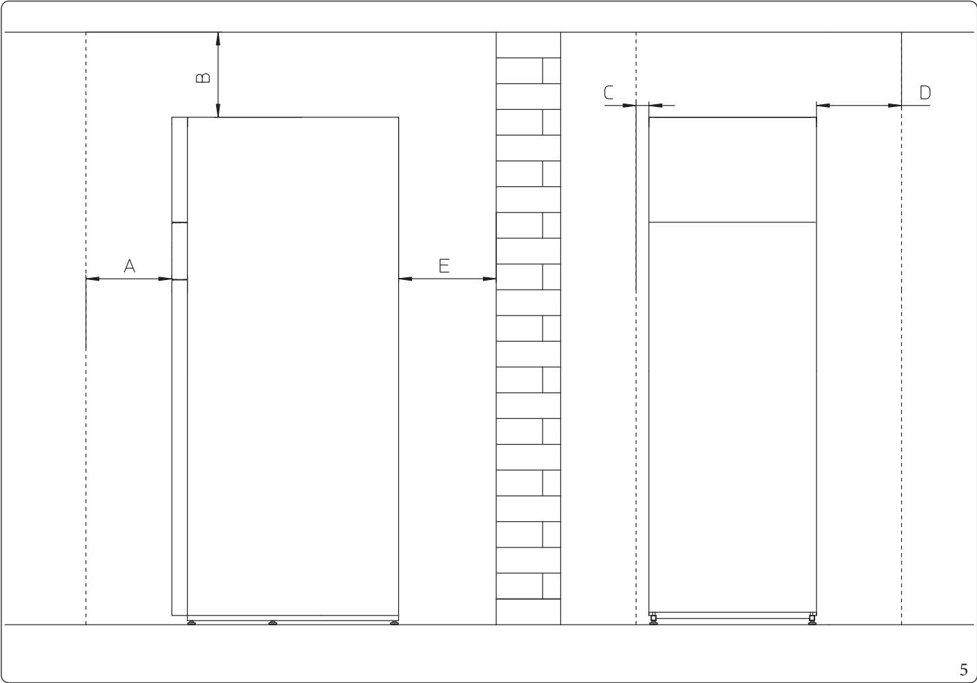
Legenda (Fig. 5): A - 450 mm B - 350 mm C - 30 mm D - 300 mm E - 10 mm
